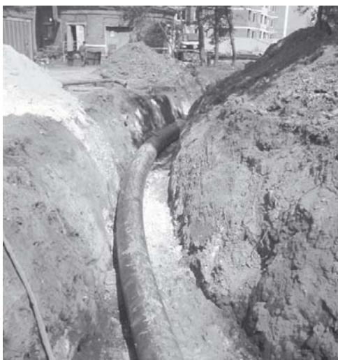
Замена напорного канализационного коллектора Д-600 от КНС 3
